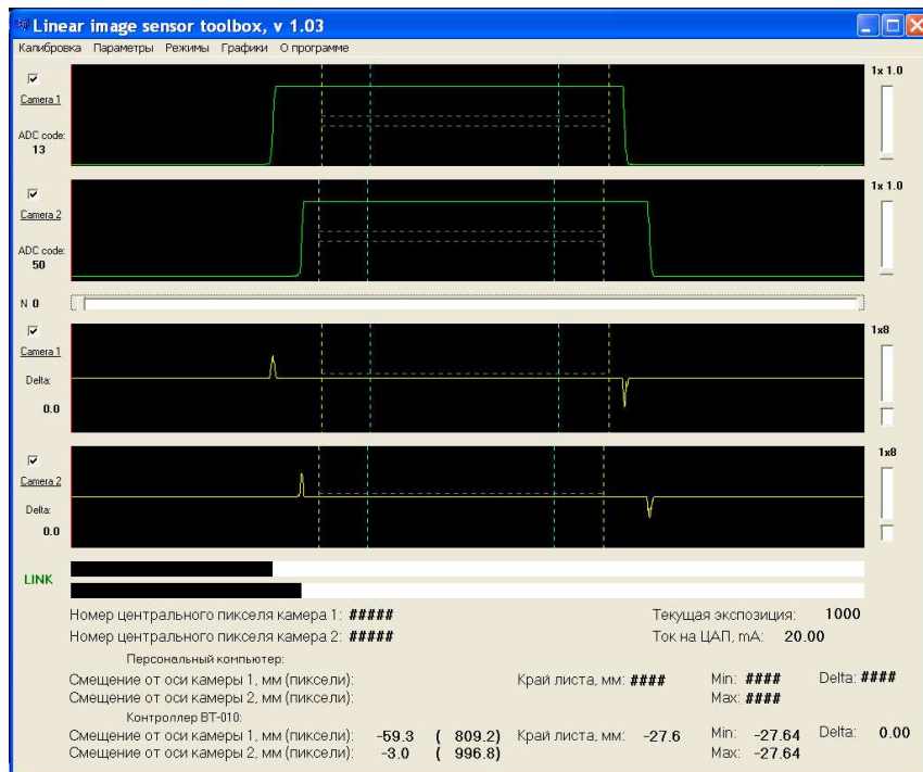
Рисунок 6 – Правильная настройка осветителя ОС
