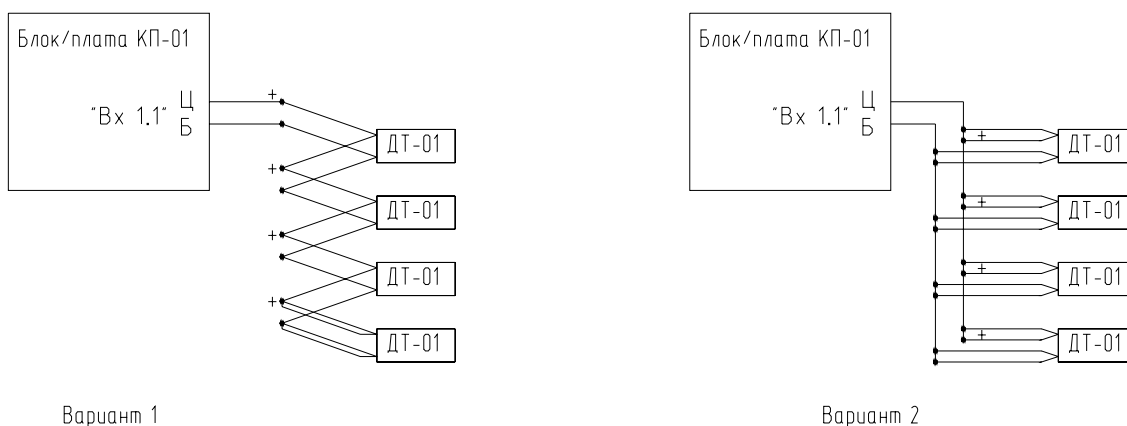
Рисунок 5 - Схема подключения датчиков температуры
