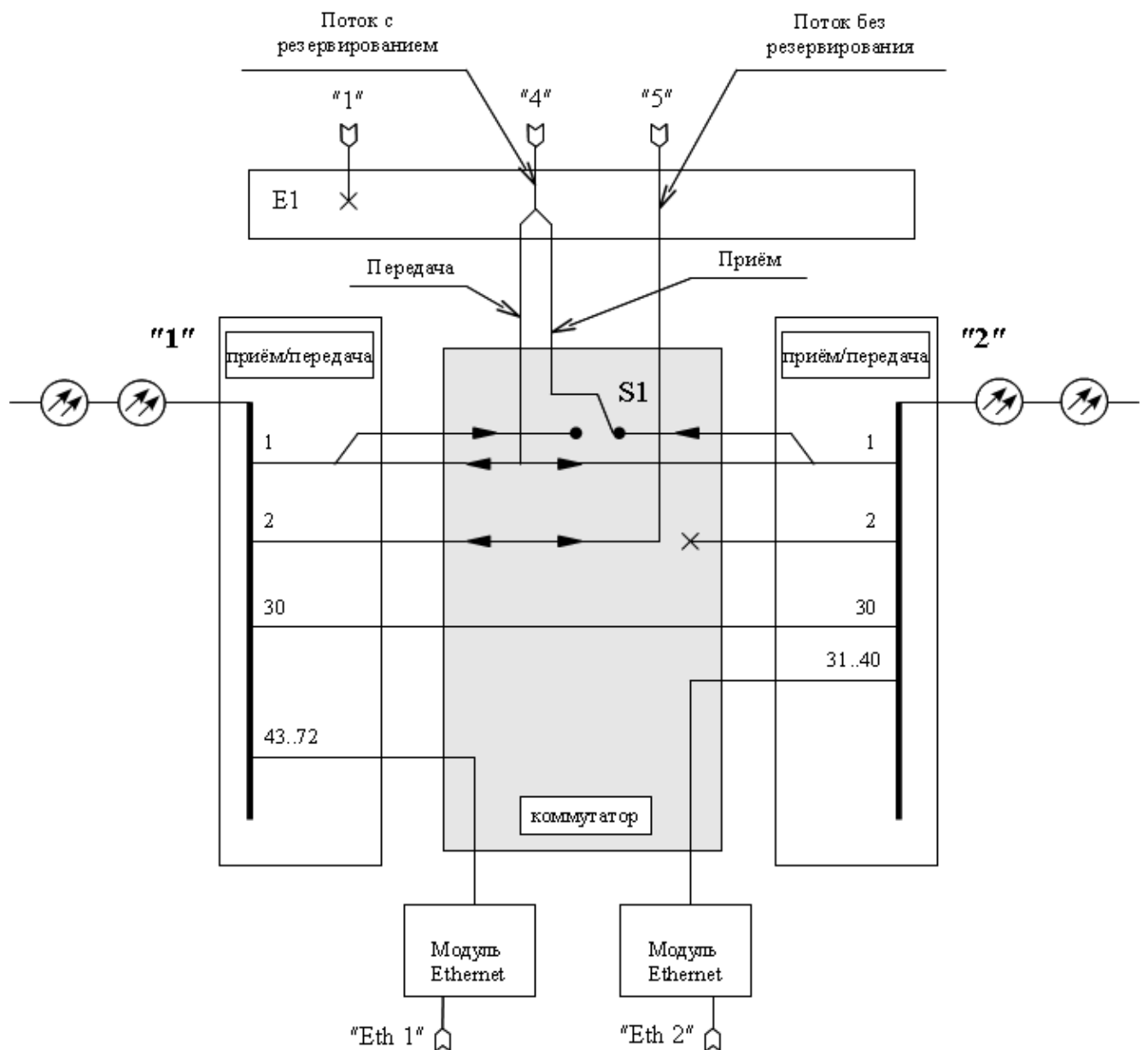
Рис. 4 Схема коммутации блока ОТ-04 в режиме «кольцо»
