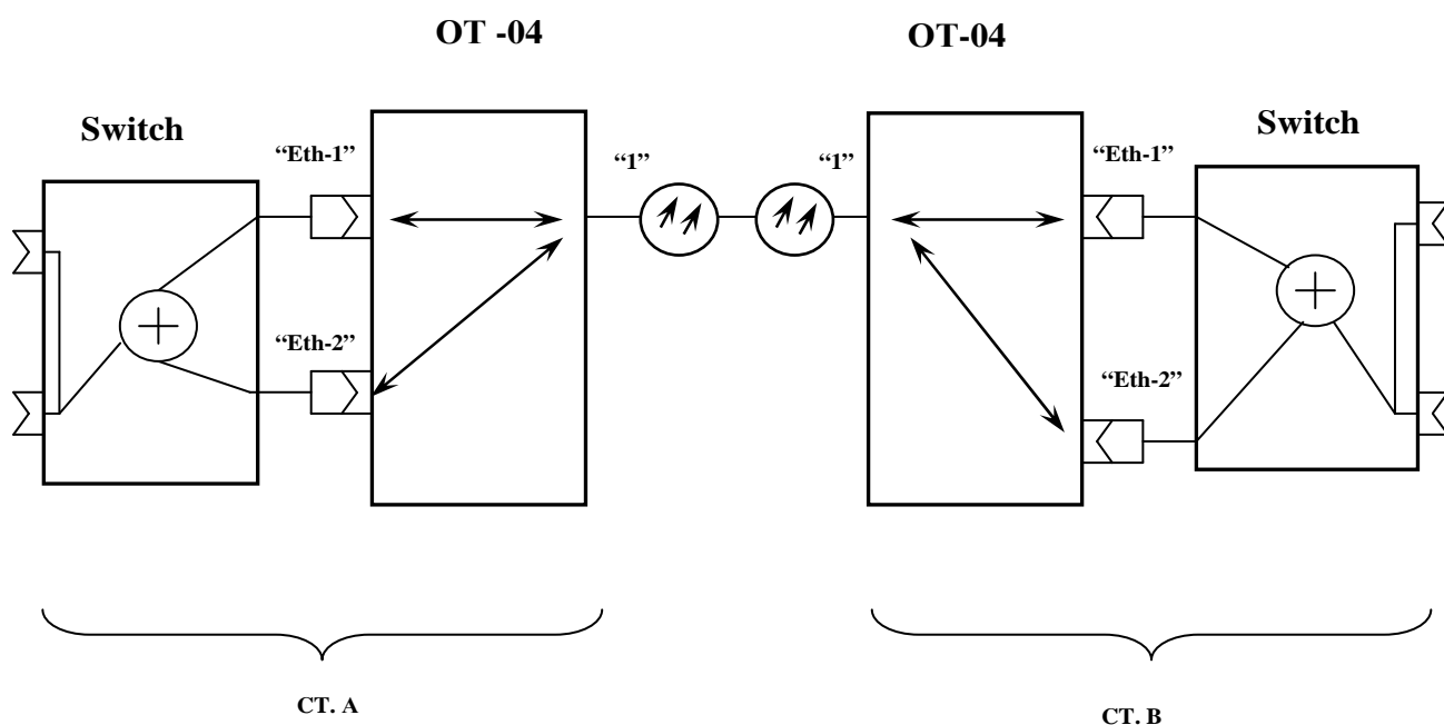
Рис. 5 Топология точка-точка
