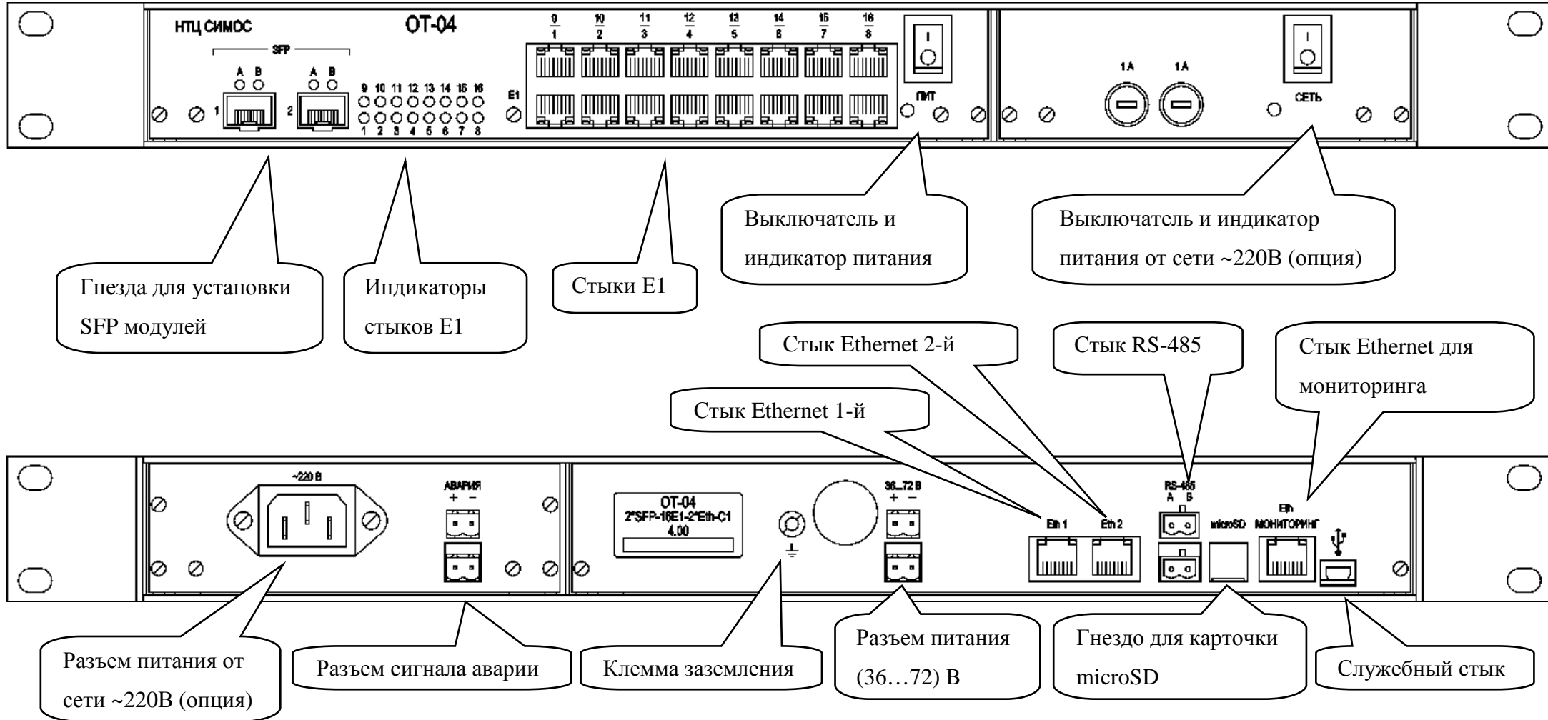
Рис. 2 Передняя (вверху) и задняя панели блока
