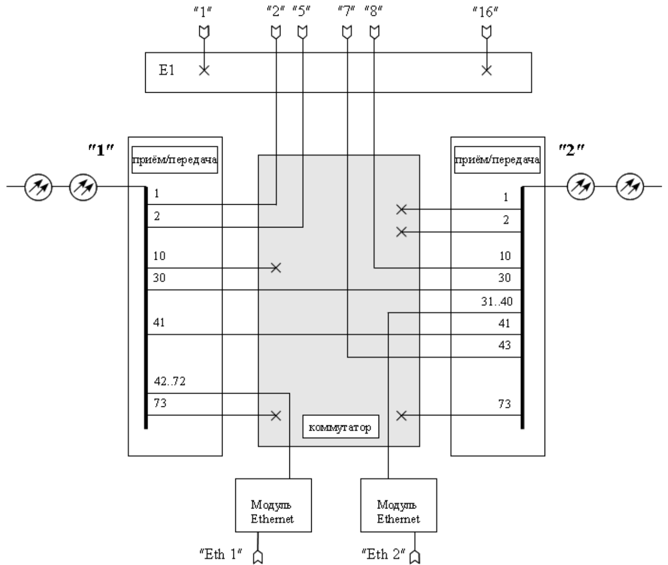
Рис. 3 Схема коммутации блока ОТ-04 в режиме «линия»
