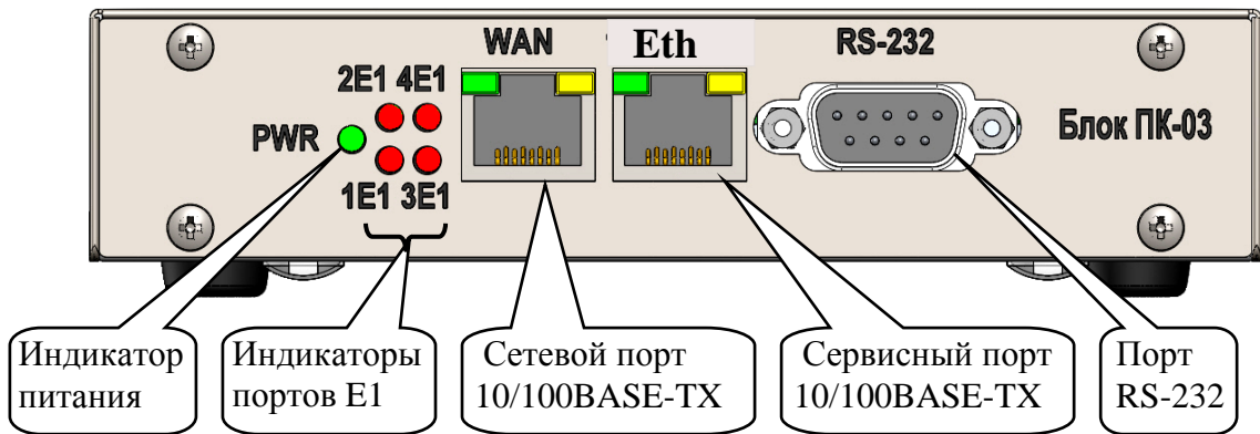
Рис. 3. Блок ПК-03. Вид спереди.
