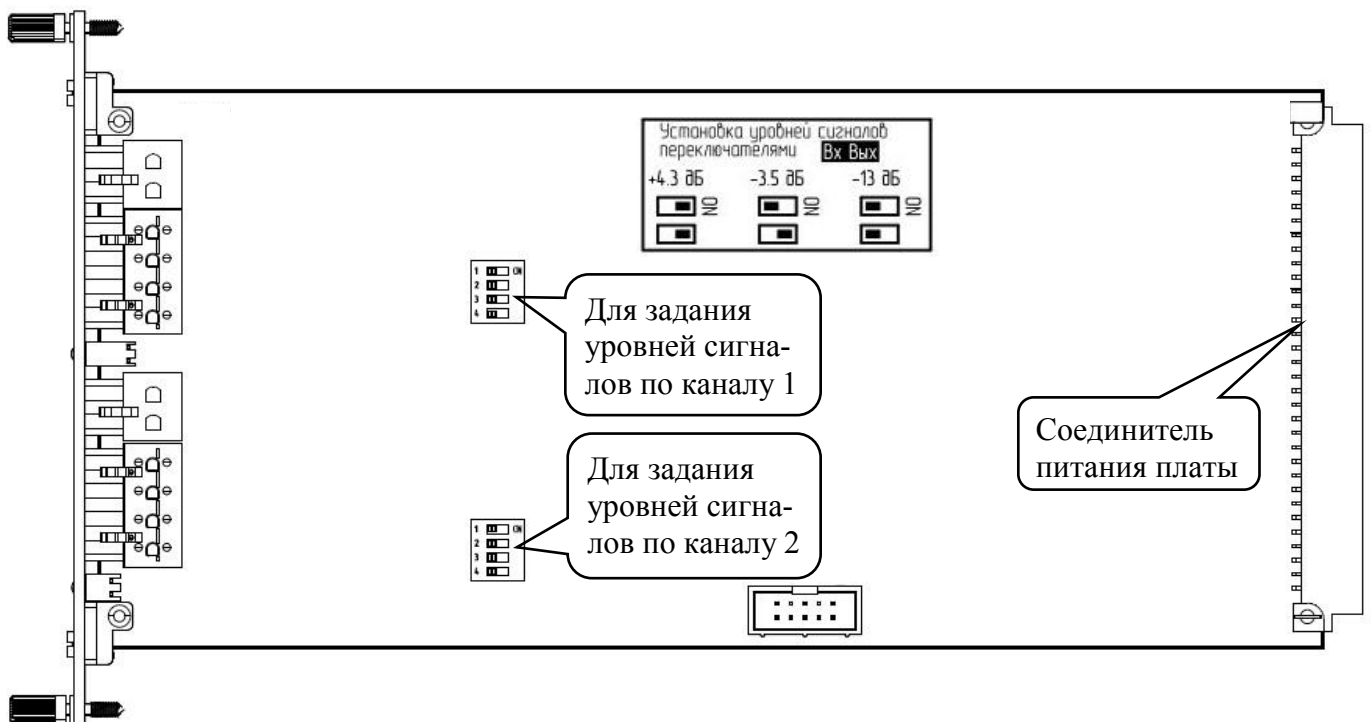
Расположение сдвиговых переключателей на плате
