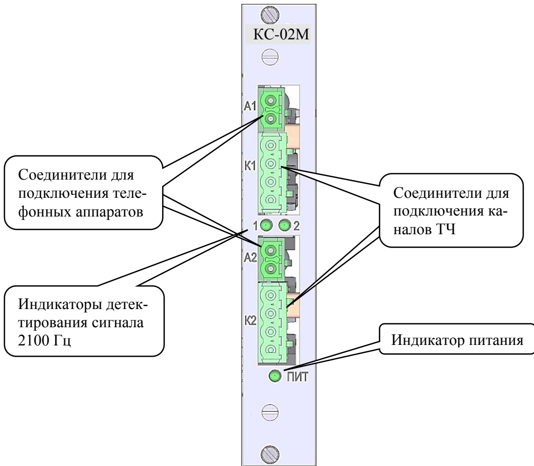
Вид платы со стороны планки
